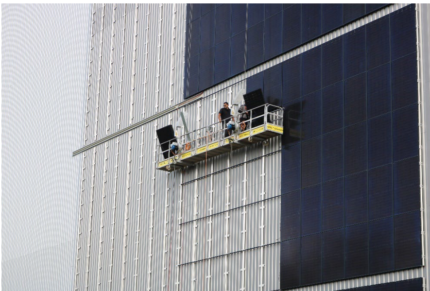
Bild 2: Photovoltaik_Installation.jpg
